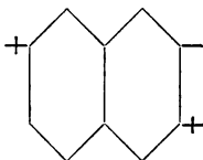
J Disulfosäure. D.R.P. 4400. Weinberg. Ber. 20. 2911.
